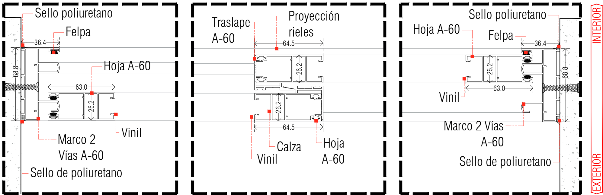
Corte A
