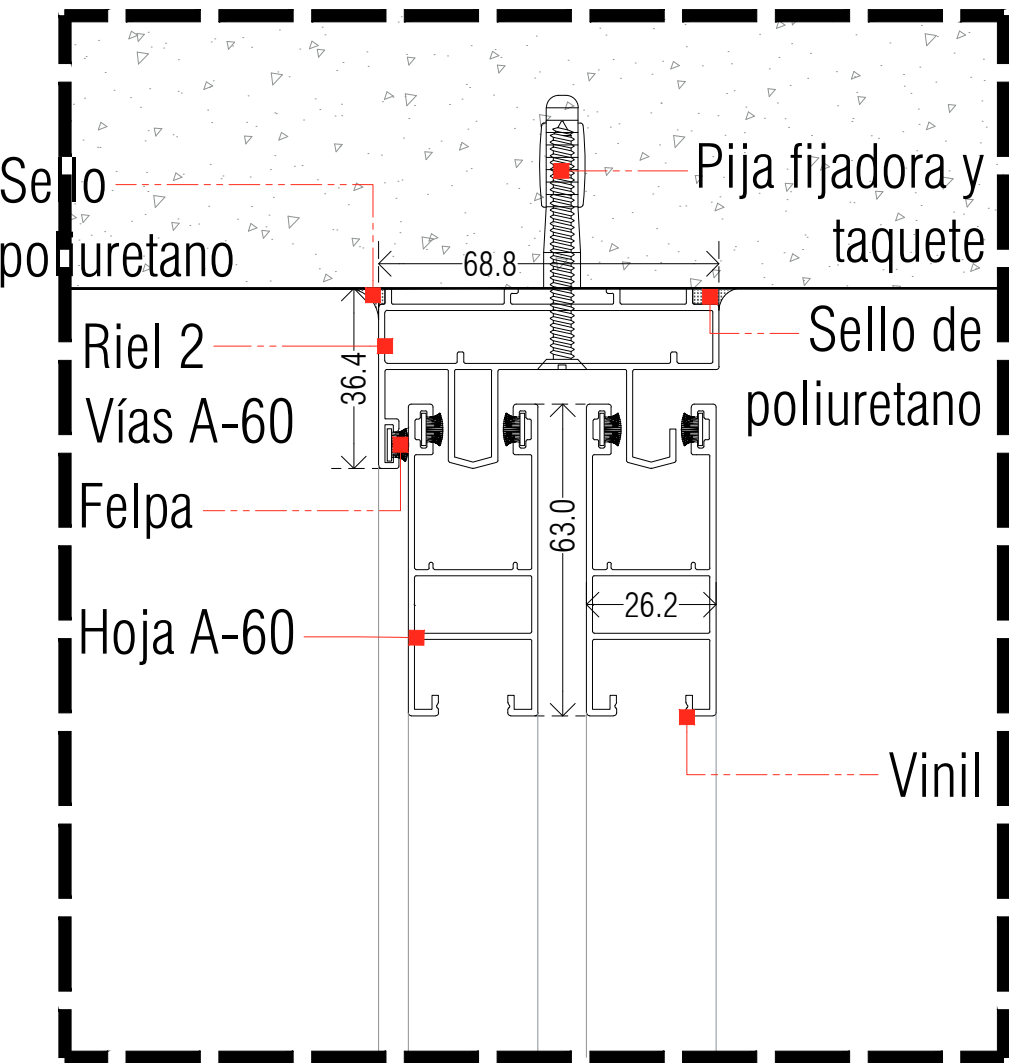
Corte B
